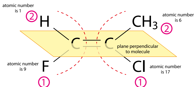
Figure 10.91 (Z)-1-fluoro-2-chloroprop-1-ene.
