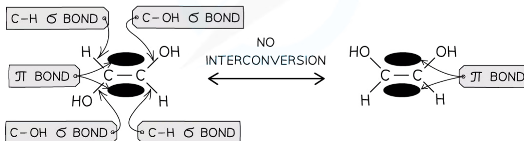
TRANS-1, 2-ETHENEDIOL
